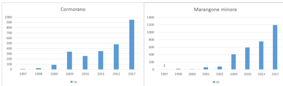
Figura 9-1 Cormorano e marangone minore: andamenti per la regione Veneto, 1997-2017.
